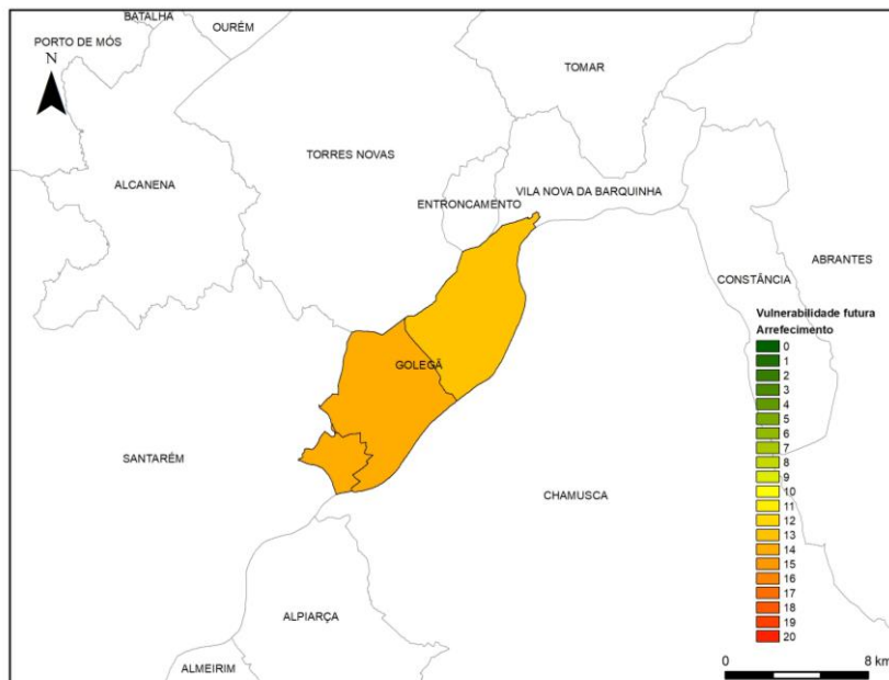
Figura 21 | Índice de vulnerabilidade futura do arrefecimento do parque edificado do município da Golegã desagregado por freguesia
